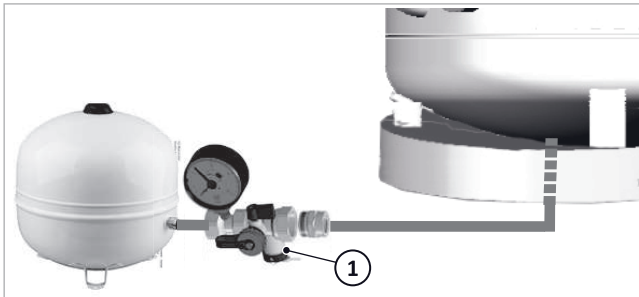
Abb. 11: KFE-Hahn an MAG-Anschlussgruppe
