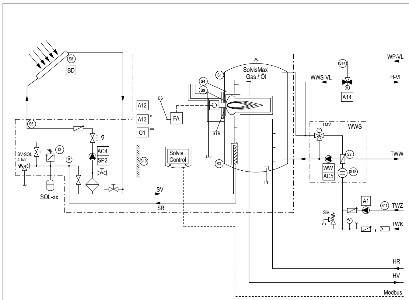
Abb. 17: SolvisMax Baureihe 6 Grundausstattung mit SC-3, SolvisLea Pro oder SolvisPia 13/17 und drei Heizkreisen – Teil 1
