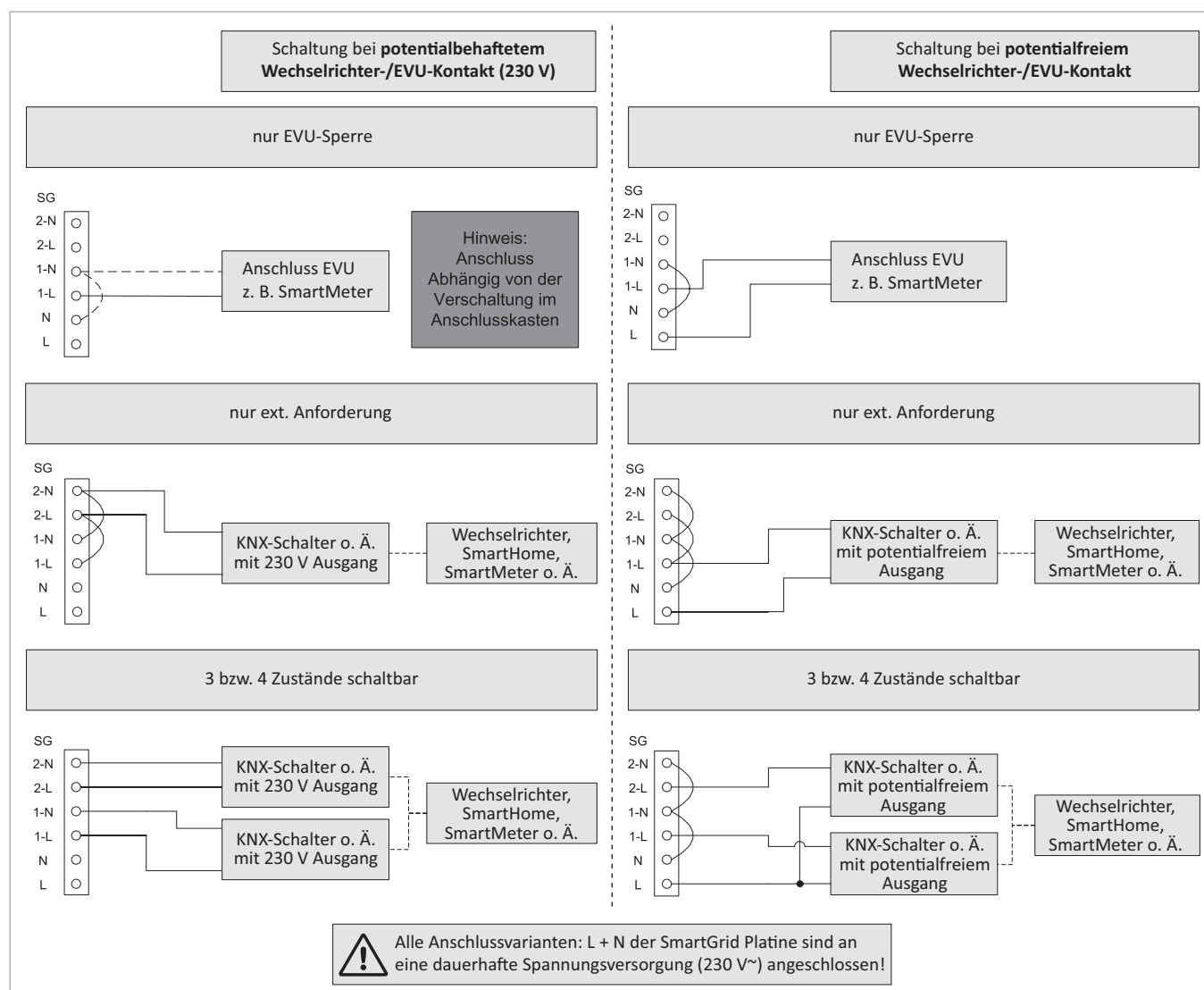
Abb. 21: Anschlussoptionen SmartGrid für die Netzplatine der SolvisControl 3
