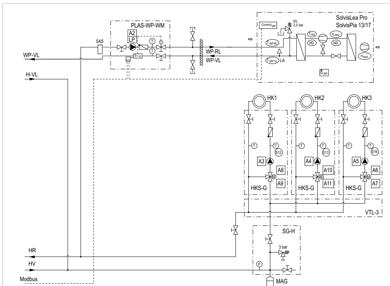
Abb. 18: SolvisMax Baureihe 6 Grundausstattung mit SC-3, SolvisLea Pro oder SolvisPia 13/17 und drei Heizkreisen – Teil 2
