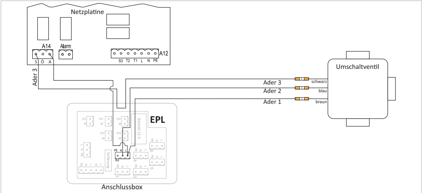
Abb. 22: Anschluss des Umschaltventils an Netz-/Erweiterungsplatine
