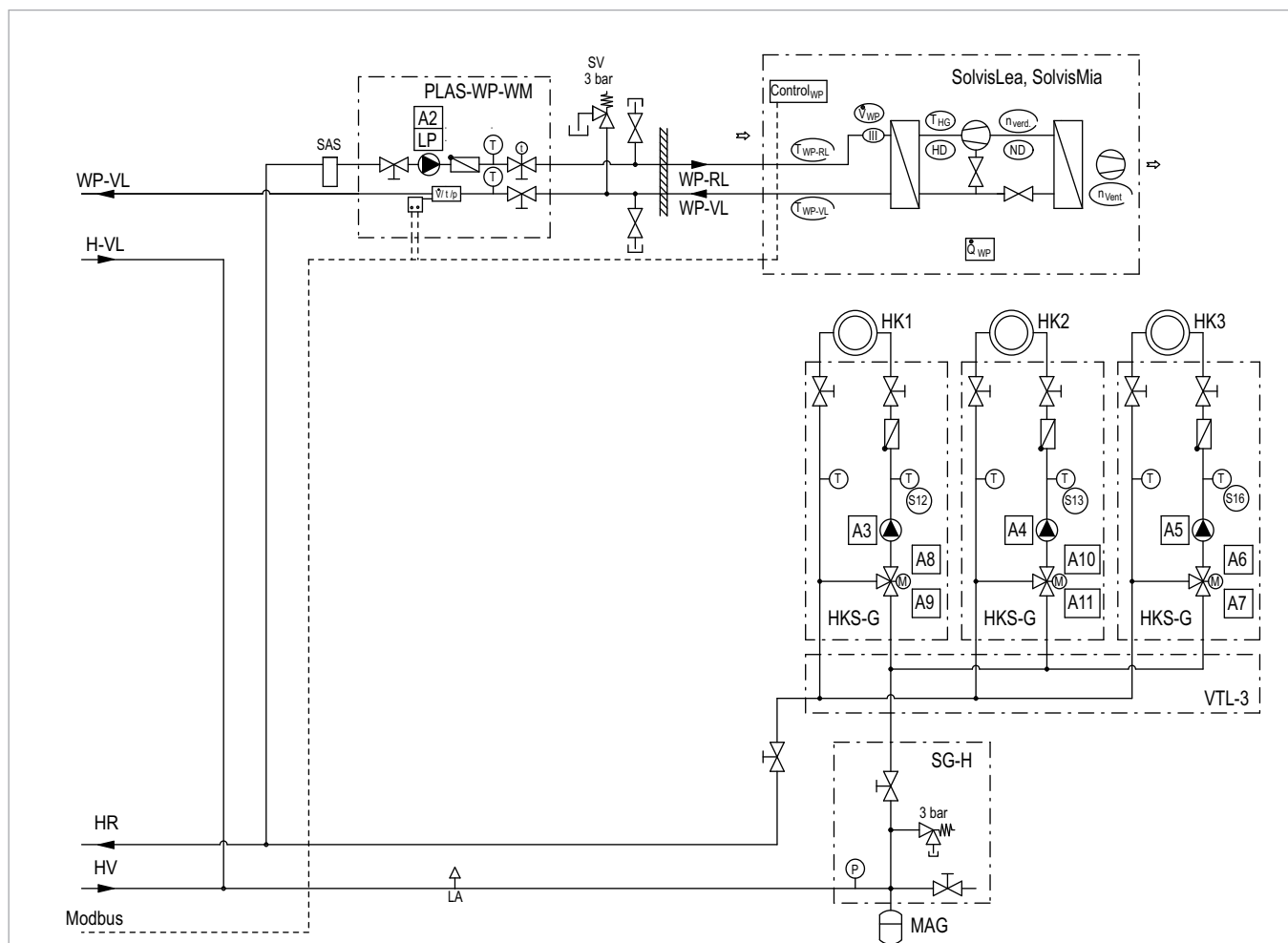
Abb. 14: SolvisMax Baureihe 6 Grundausstattung mit SC-3, SolvisLea/SolvisMia und drei Heizkreisen – Teil 2
