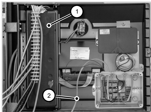
Abb. 10: Anschluss Umschaltventil
