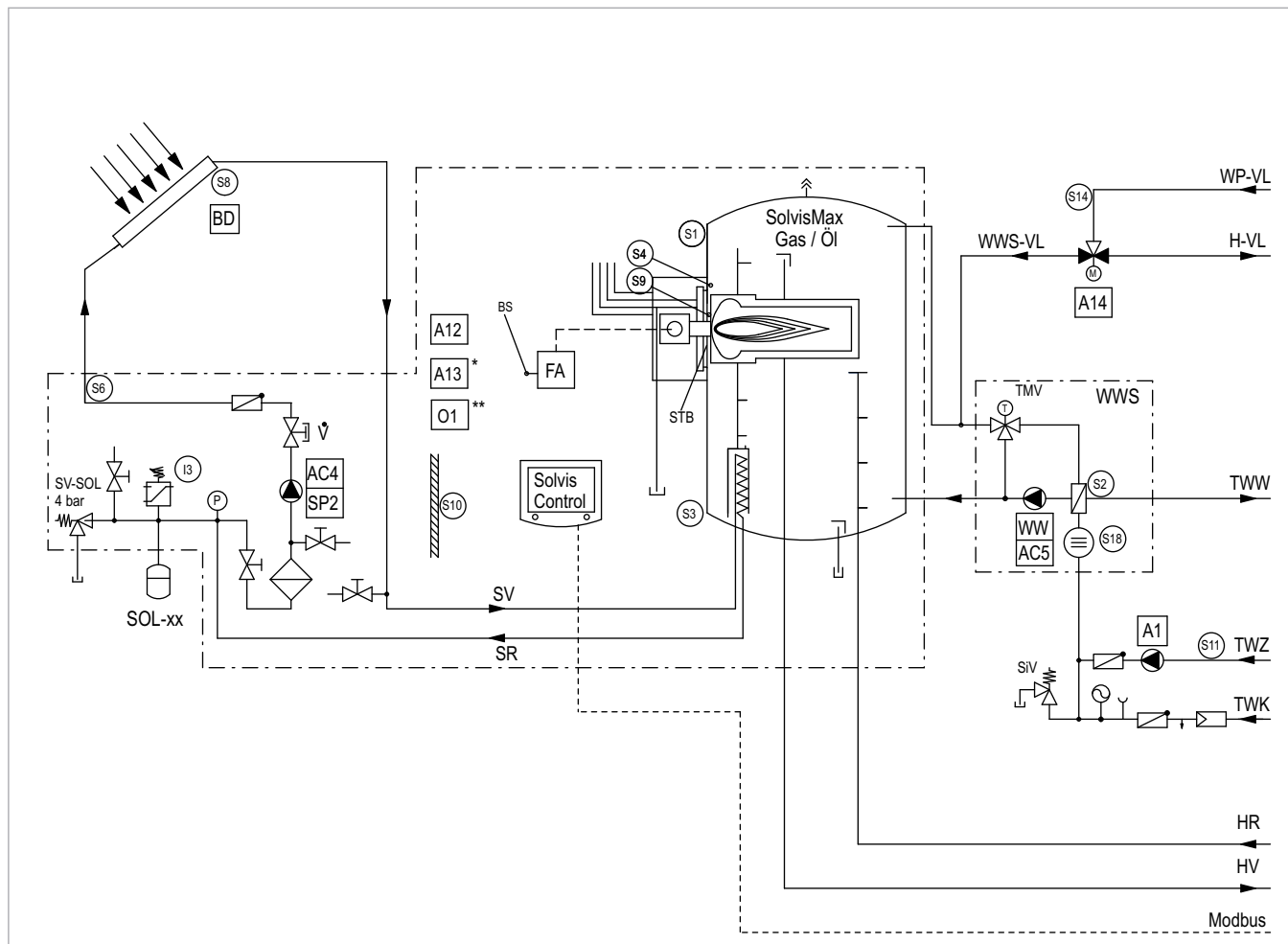
Abb. 13: SolvisMax Baureihe 6 Grundausstattung mit SC-3, SolvisLea/SolvisMia und drei Heizkreisen – Teil 1
