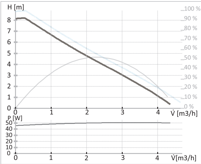
Abb. 12: Pumpenkennlinie IMP NMT Mini PWM 15/80-130 (konstante Drehzahl)
