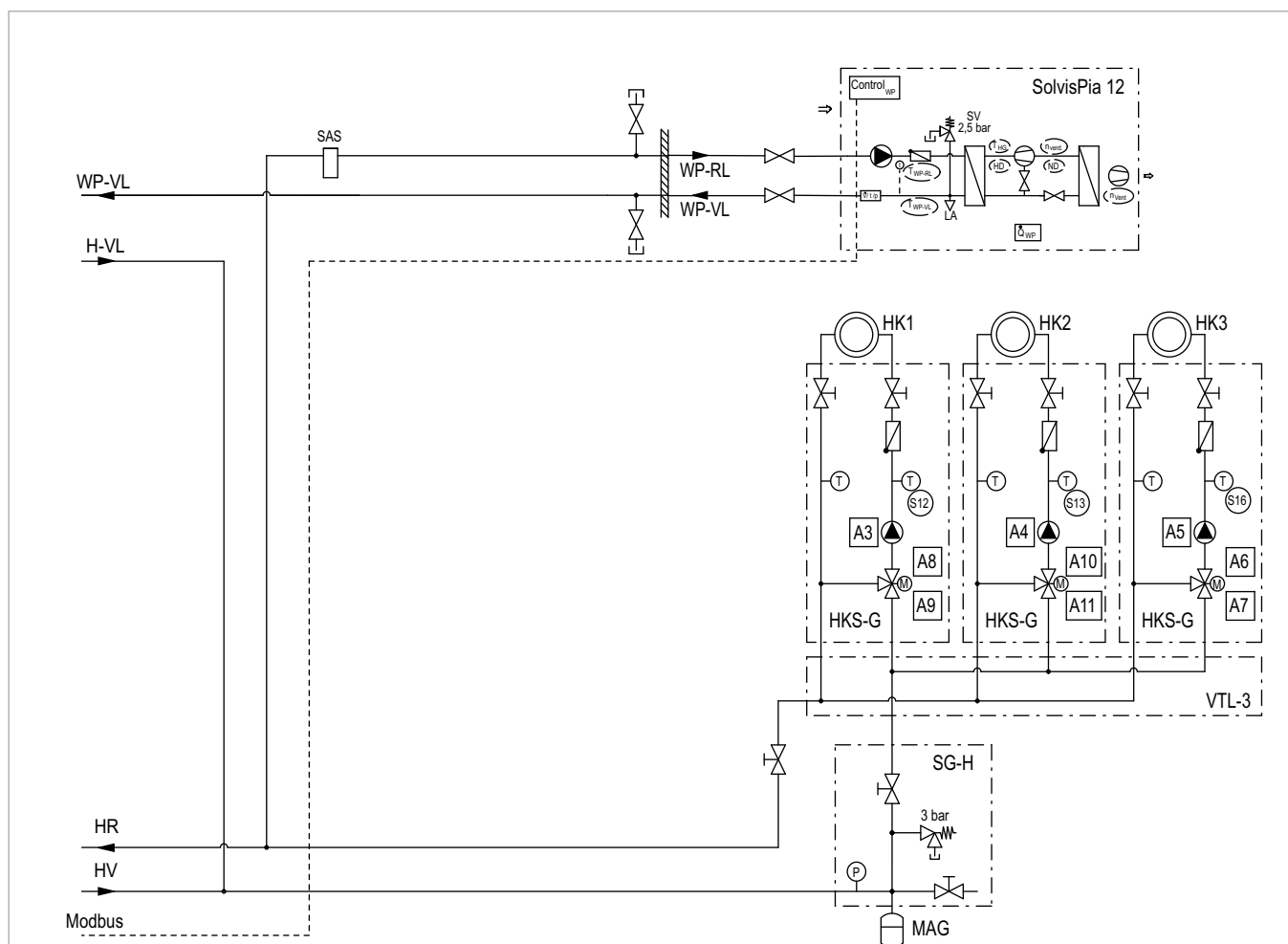
Abb. 16: SolvisMax Baureihe 6 Grundausstattung mit SC-3, SolvisPia 12 und drei Heizkreisen – Teil 2
