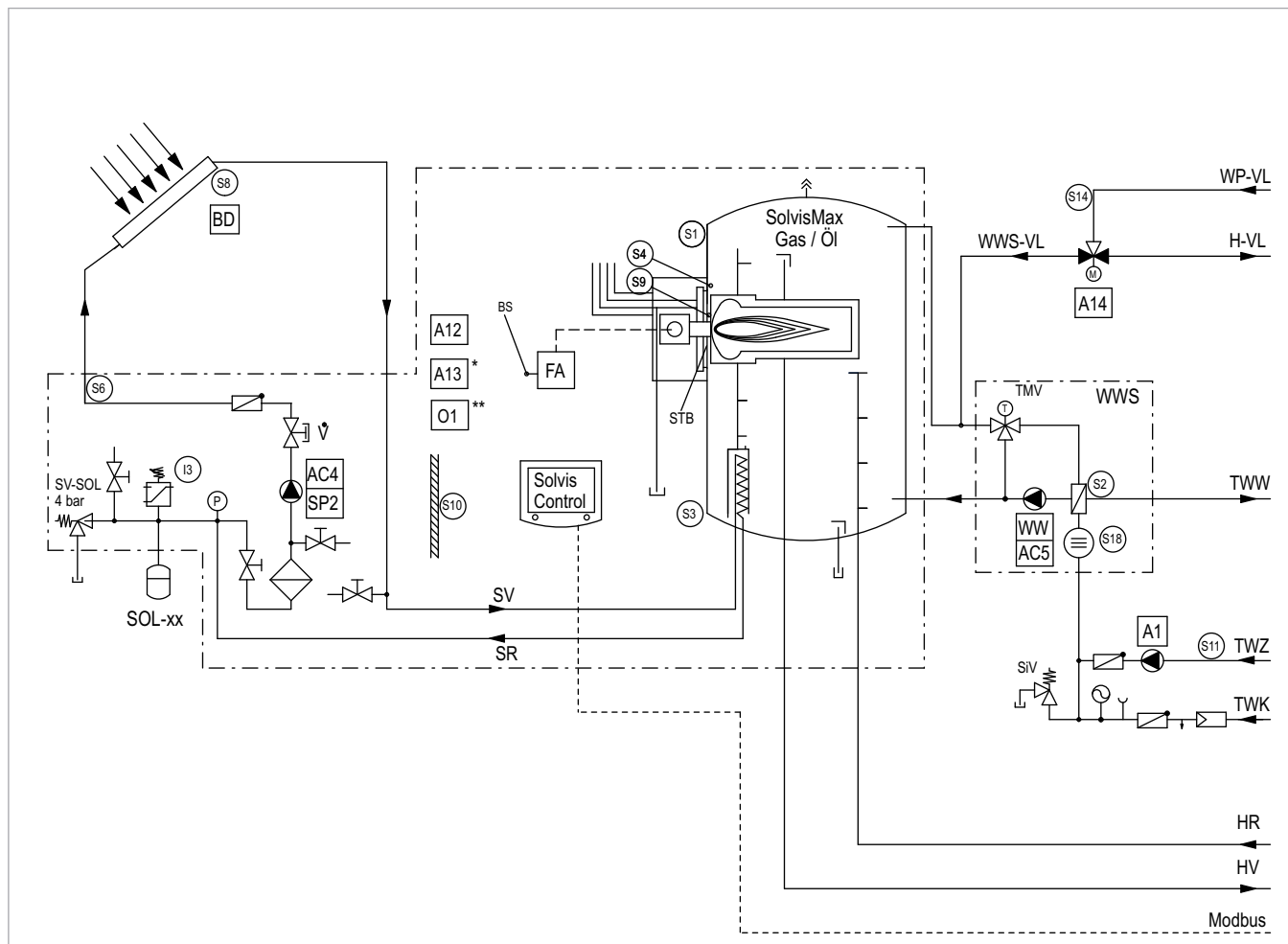
Abb. 15: SolvisMax Baureihe 6 Grundausstattung mit SC-3, SolvisPia 12 und drei Heizkreisen – Teil 1
