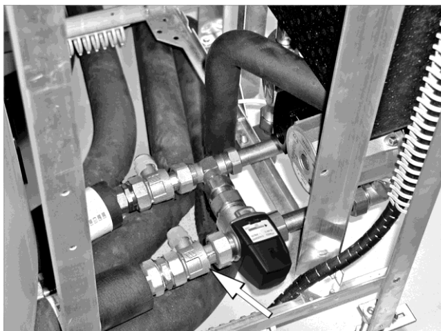
Abb. 3: Anschlussposition am Warmwasservorlauf des SolvisMax 6
