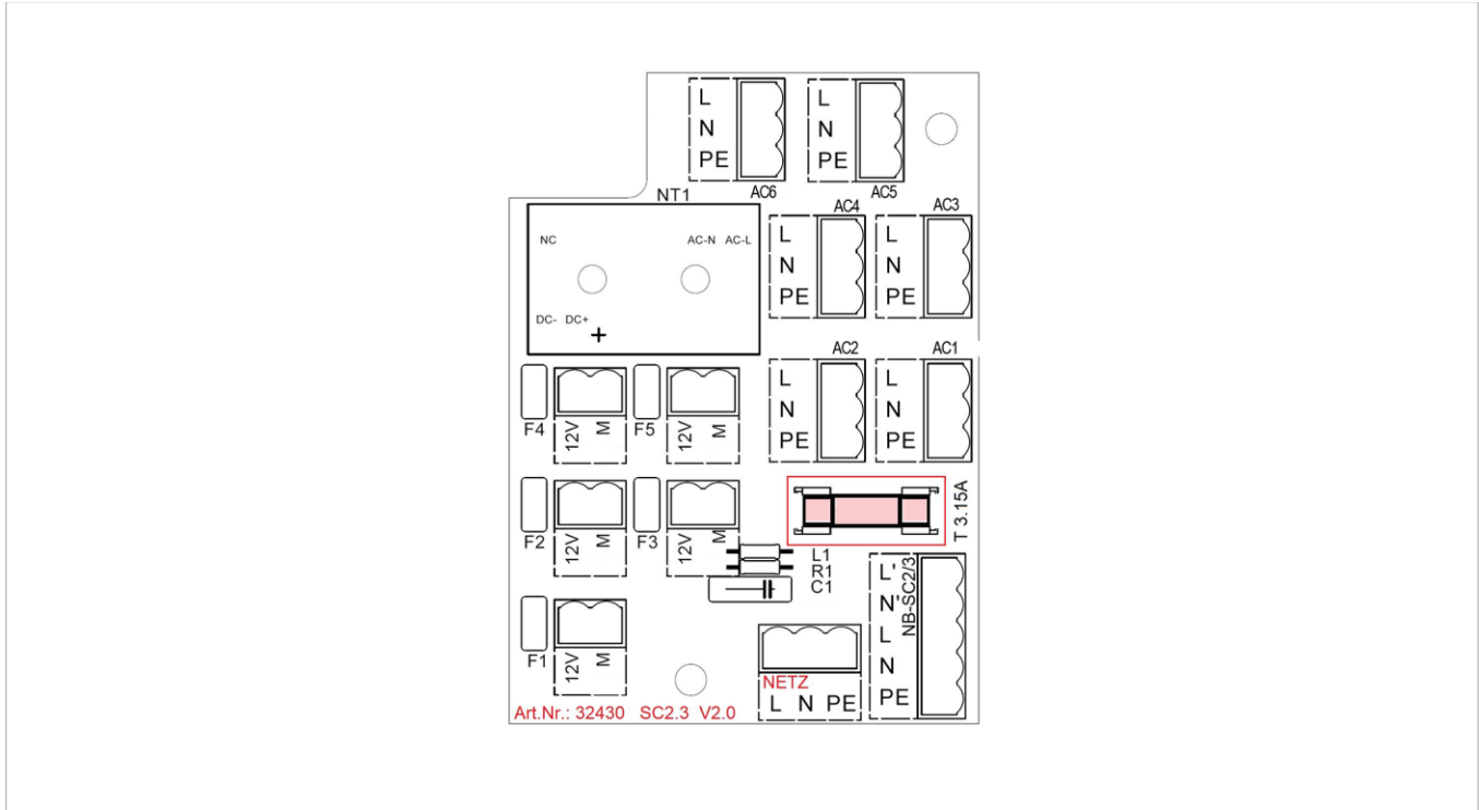
Abb. 20: Erweiterungsplatine für die Netzplatine der SolvisControl 3
