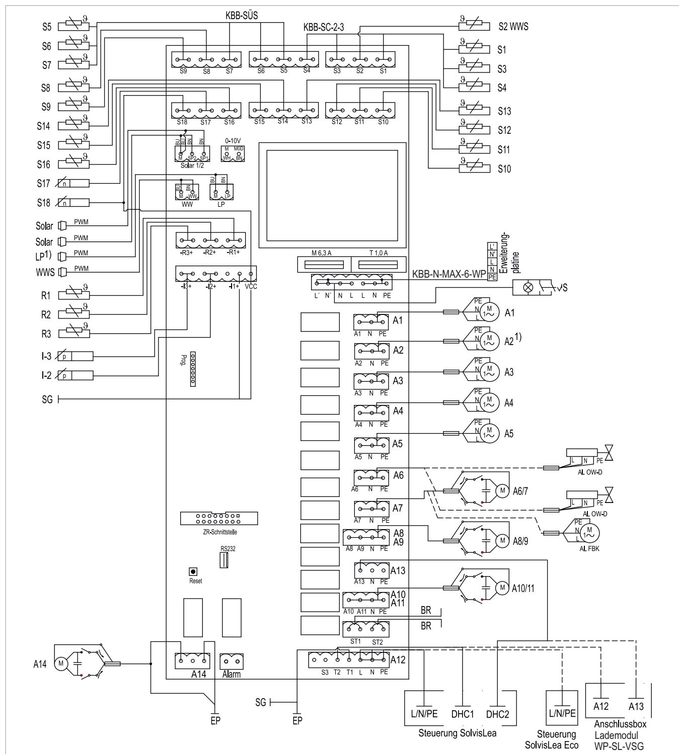
Abb. 19: Netzplatine SolvisControl 3 für SolvisMax 6 Gas-/Öl-Hybrid mit SolvisMia / SolvisLea / Lea Eco / SolvisPia
