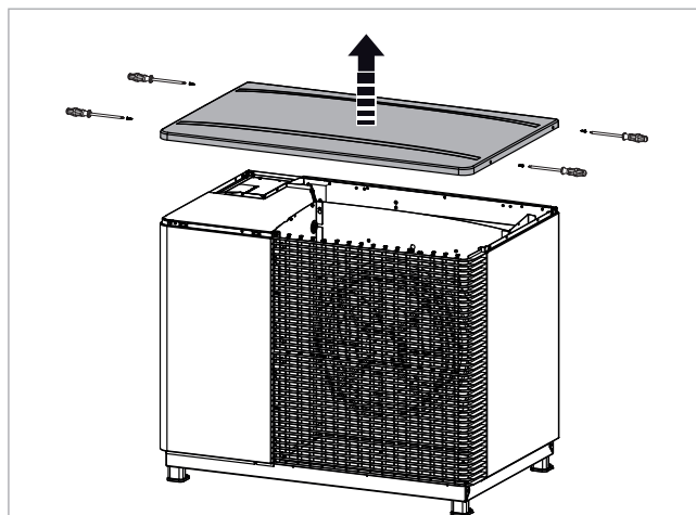
Abb. 1: Deckel von SolvisLea 7 Pro entfernen
