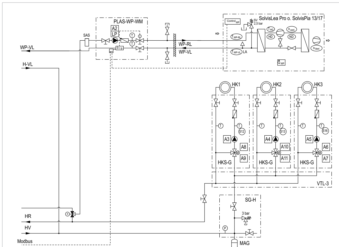
Abb. 7: SolvisMax Baureihe 6 Grundausstattung mit SC-3, Hydraulikset SmartGrid, SolvisLea Pro oder SolvisPia 13/17 und drei Heizkreisen – Teil 2
