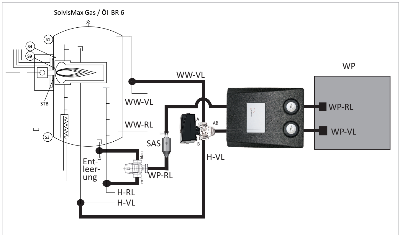
Abb. 4: Anschluss des Hydrauliksets SmartGrid in schematischer Darstellung
