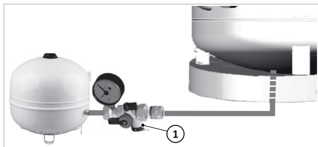
Abb. 5: KFE-Hahn an MAG-Anschlussgruppe
