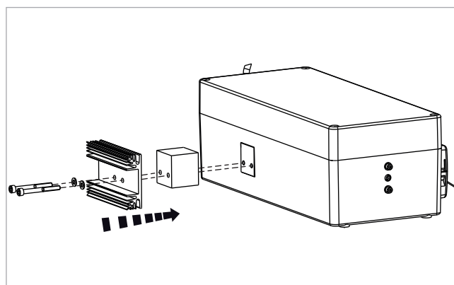
Abb. 1: Kühlkörper mit Verlängerungselement montieren
